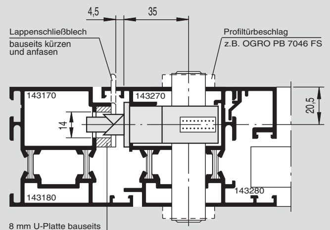
SCHÜCO Iskotherm 74 mit DORMA SVP xx19
